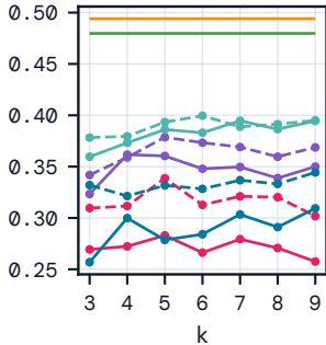
MAE (%)
